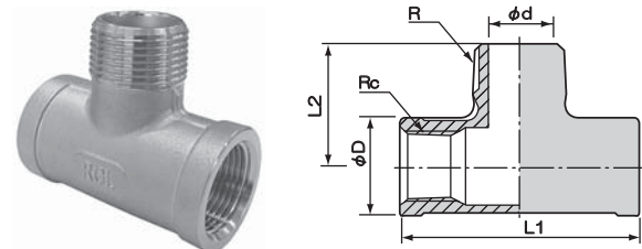
型式:R-2F 単位:mm
