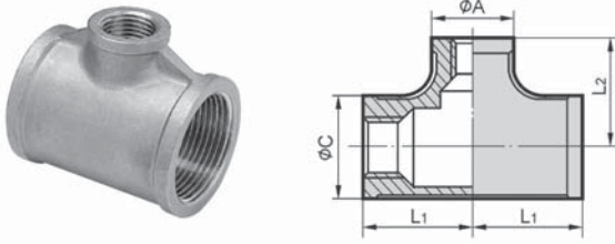
型式:R-2A 単位:mm
