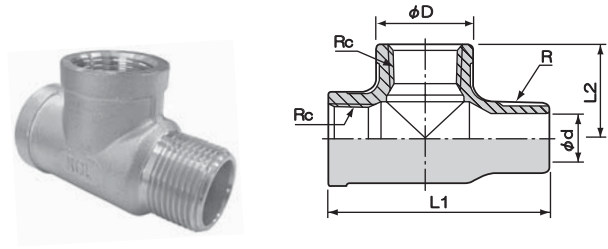
型式:R-2E 単位:mm
