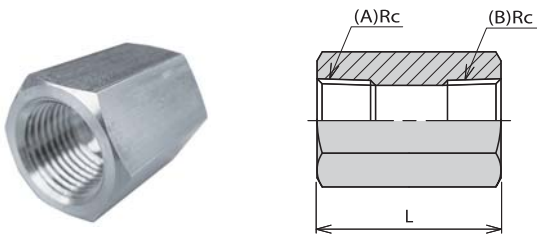
型式:RH-12K 単位:mm
