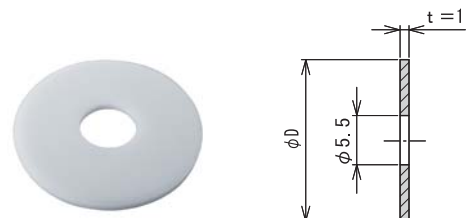
型式:RH-18P 単位:mm
