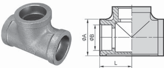
型式:R-2B 単位:mm
