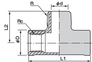
型式:R-2F 単位:mm
