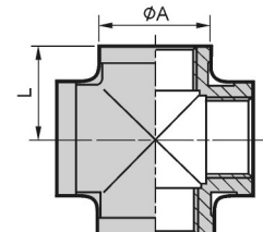
型式:R-3 単位:mm
