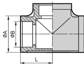
型式:R-2B 単位:mm
