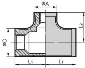
型式:R-2A 単位:mm
