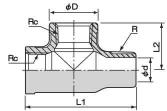
型式:R-2E 単位:mm
