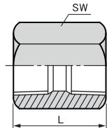
型式:R-12K 単位:mm
