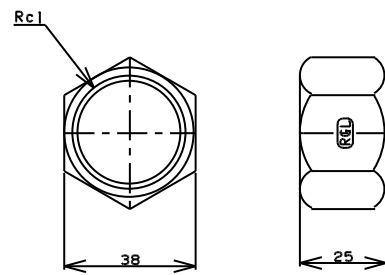
TITLE 六角キャップ MODEL R-10-1
