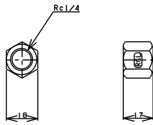
TITLE 六角キャップ MODEL R-10-1/4
