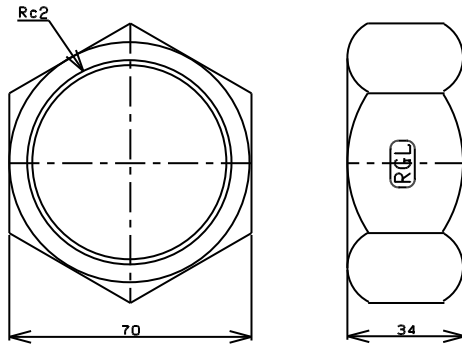
TITLE 六角キャップ MODEL R-10-2
