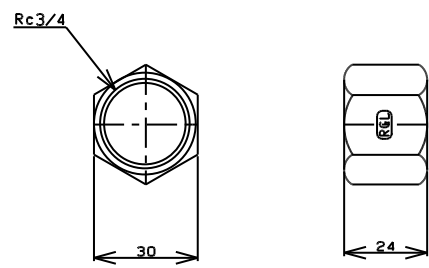
TITLE 六角キャップ MODEL R-10-3/4
