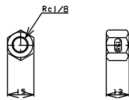
TITLE 六角キャップ MODEL R-10-1/8
