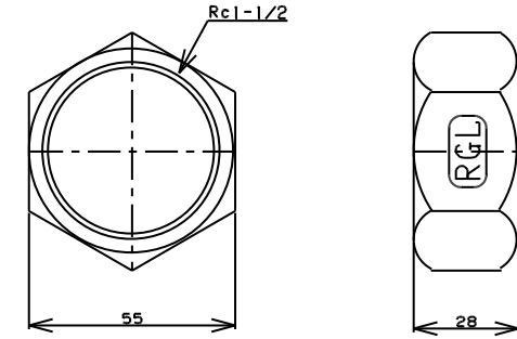
TITLE 六角キャップ MODEL R-10-1/2
