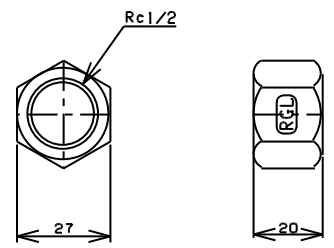
TITLE 六角キャップ MODEL R-10-1/2
