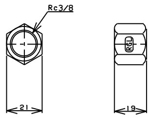
TITLE 六角キャップ MODEL R-10-3/8
