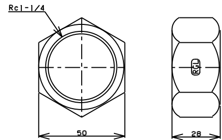
TITLE 六角キャップ MODEL R-10-1-1/4
