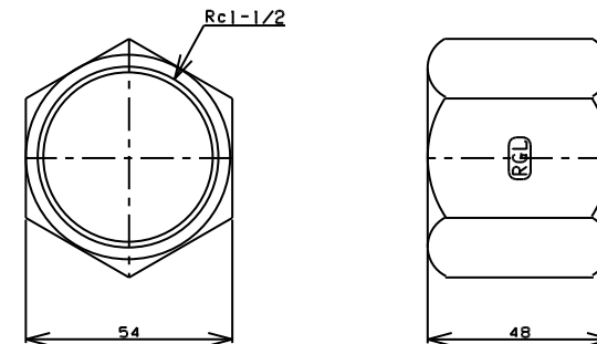
TITLE 六角ソケット MODEL R-12K-1-1/2
