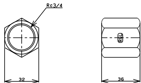
TITLE 六角ソケット MODEL R-12K-3/4
