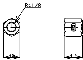
TITLE 六角ソケット MODEL R-12K-1/8
