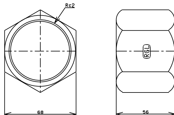
TITLE 六角ソケット MODEL R-12K-2
