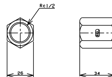
TITLE 六角ソケット MODEL R-12K-1/2
