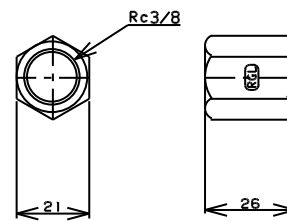
TITLE 六角ソケット MODEL R-12K-3/8
