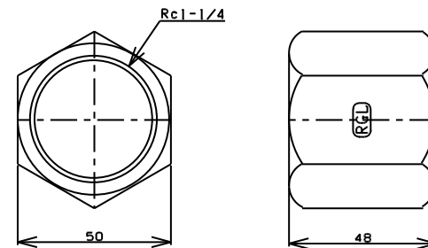
TITLE 六角ソケット MODEL R-12K-1-1/4
