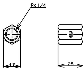
TITLE 六角ソケット MODEL R-12K-1/4
