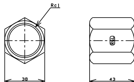
TITLE 六角ソケット MODEL R-12K-1
