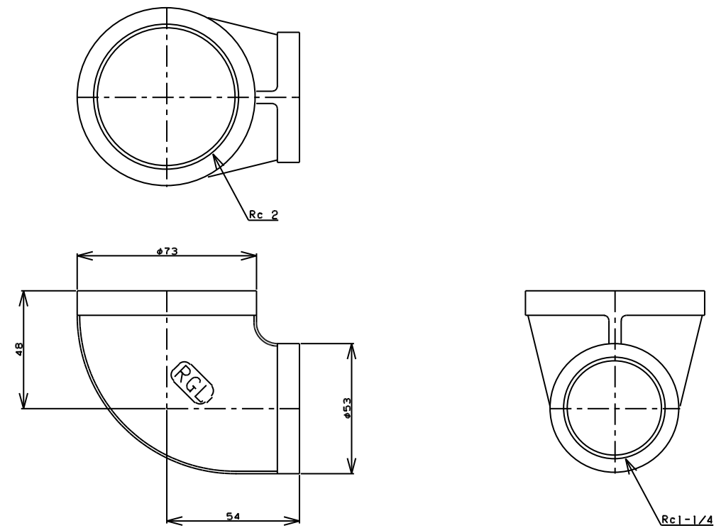
TITLE 径違い90°エルボ MODEL R-1A-2X1-1/4
