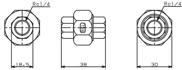
TITLE ヌヌヌヌニオン (PTFEガスケット) MODEL R-6A-1/4
