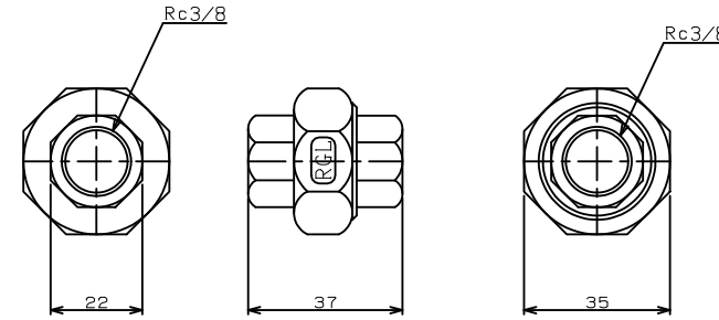
TITLE ヌヌヌヌニオン (PTFEガスケット) MODEL R-6A-3/8
