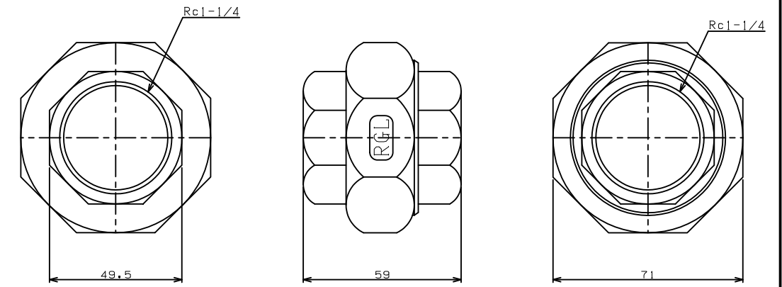
TITLE ヌヌヌヌニオン (PTFEガスケット) MODEL R-6A-1-1/4
