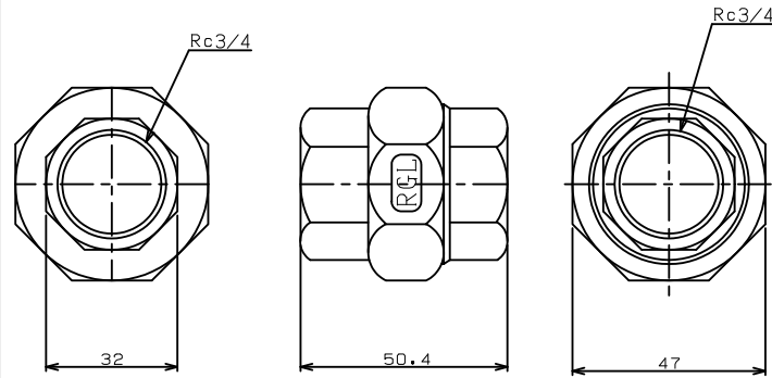
TITLE ヌヌヌヌニオン (PTFEガスケット) MODEL R-6A-3/4
