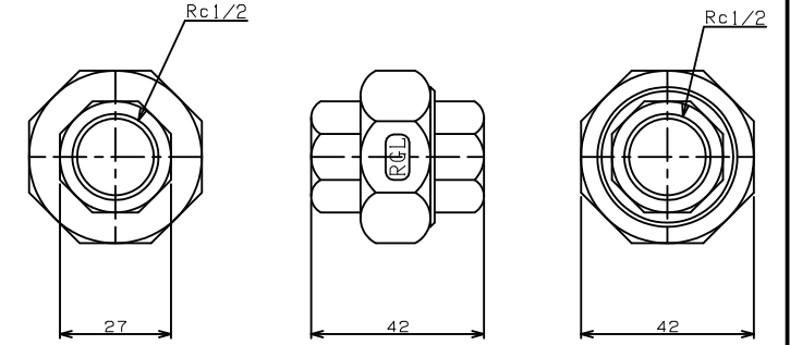
TITLE ヌヌヌヌニオン (PTFEガスケット) MODEL R-6A-1/2
