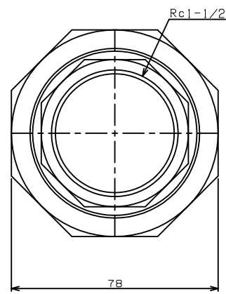
TITLE ヌヌヌヌニオン (PTFEガスケット) MODEL R-6A-1-1/2
