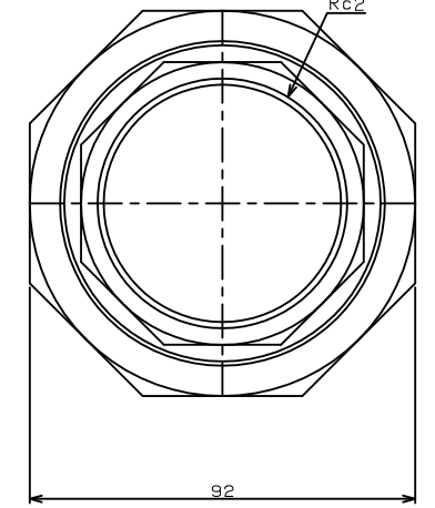
TITLE ヌヌヌヌニオン (PTFEガスケット) MODEL R-6A-2
