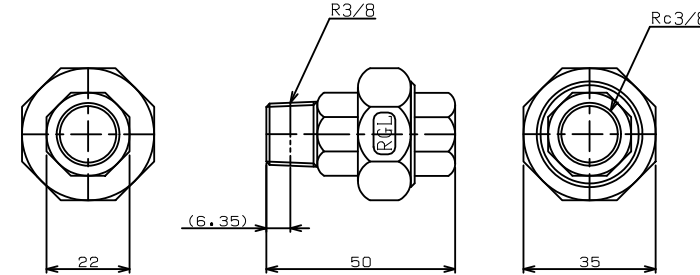
TITLE オス×メスユニオン (PTFEガスケット) MODEL R-6C-3/8
