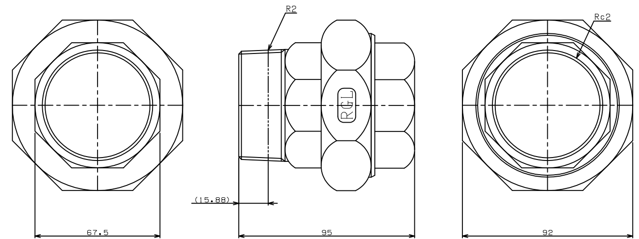
TITLE オス×メスユニオン (PTFEガスケット) MODEL R-6C-2
