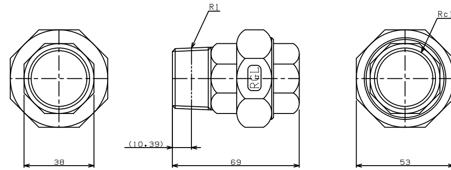
TITLE オス×メスユニオン (PTFEガスケット) MODEL R-6C-1
