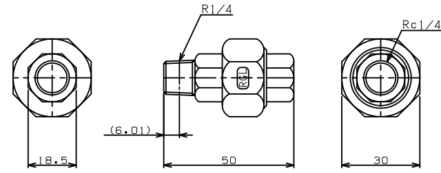
TITLE オス×メスユニオン (PTFEガスケット) MODEL R-6C-1/4
