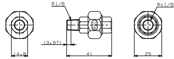
TITLE オス×メスユニオン (PTFEガスケット) MODEL R-6C-1/8
