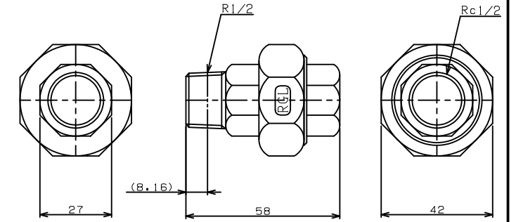
TITLE オス×メスユニオン (PTFEガスケット) MODEL R-6C-1/2
