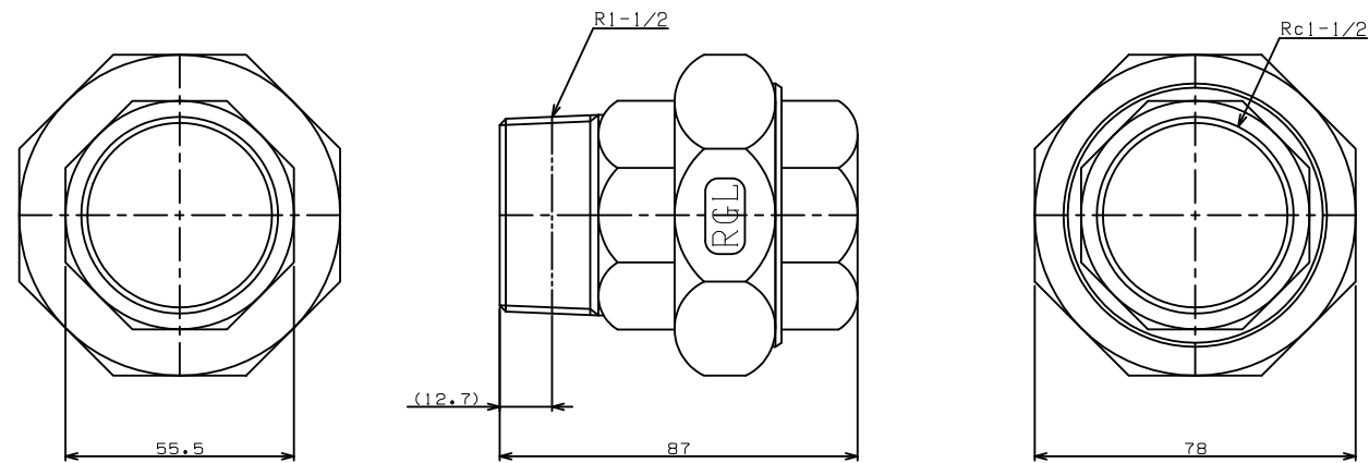
TITLE オス×メスユニオン (PTFEガスケット) MODEL R-6C-1-1/2
