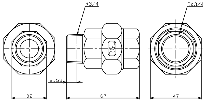
TITLE オス×メスユニオン (PTFEガスケット) MODEL R-6C-3/4
