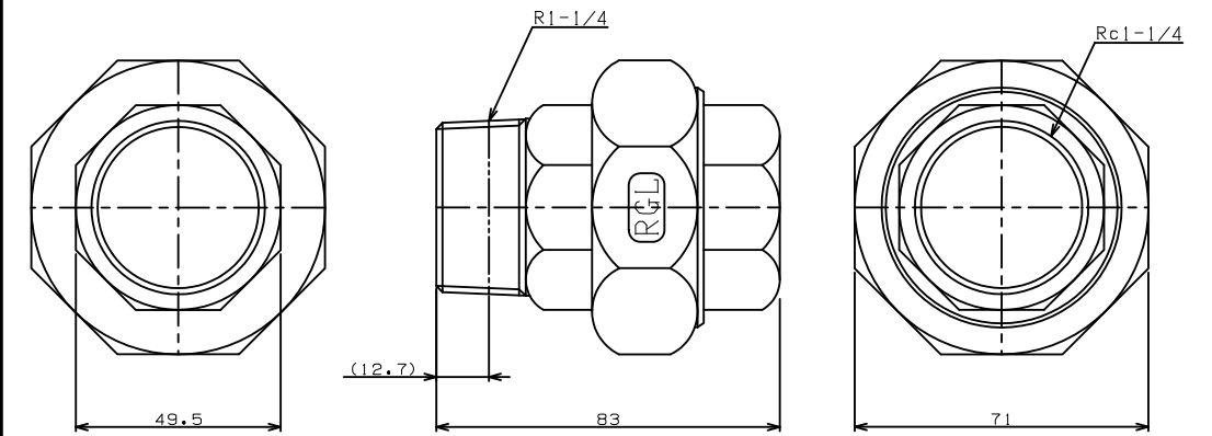
TITLE オス×メスユニオン (PTFEガスケット) MODEL R-6C-1-1/4
