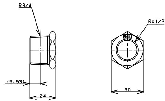
TITLE ブッシング MODEL R-9-3/4x1/2
