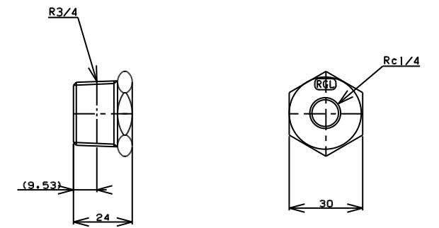
TITLE ブッシング MODEL R-9-3/4x1/4
