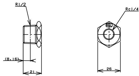
TITLE ブッシング MODEL R-9-1/2x1/4
