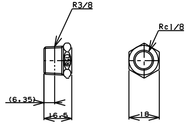
TITLE ブッシング MODEL R-9-3/8x1/8
