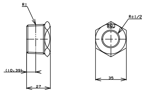
TITLE ブッシング MODEL R-9-1x1/2
