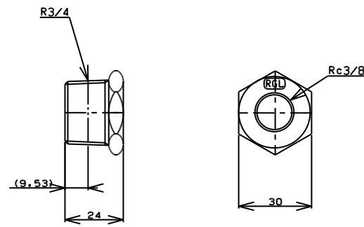
TITLE ブッシング MODEL R-9-3/4x3/8
