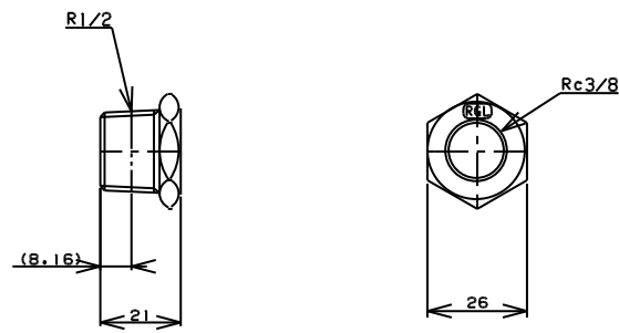
TITLE ブッシング MODEL R-9-1/2x3/8
