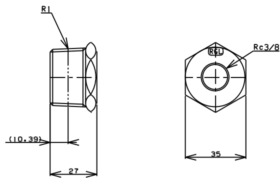
TITLE ブッシング MODEL R-9-1x3/8
