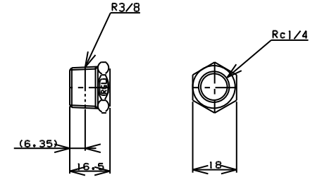
TITLE ブッシング MODEL R-9-3/8x1/4
