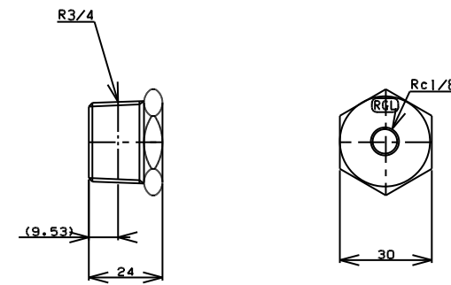
TITLE ブッシング MODEL R-9-3/4x1/8
