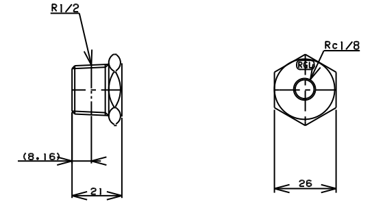
TITLE ブッシング MODEL R-9-1/2x1/8
