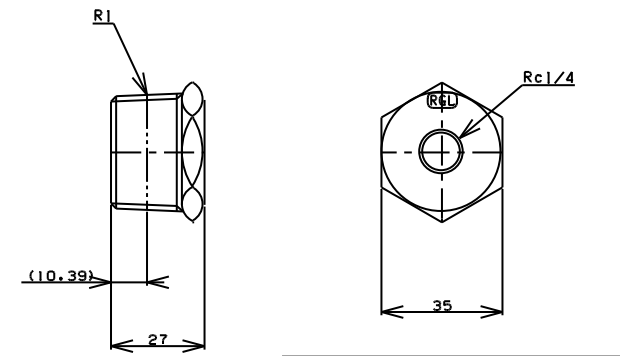
TITLE ブッシング MODEL R-9-1x1/4
