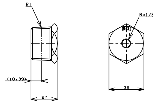
TITLE ブッシング MODEL R-9-1x1/8
