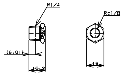
TITLE ブッシング MODEL R-9-1/4x1/8
