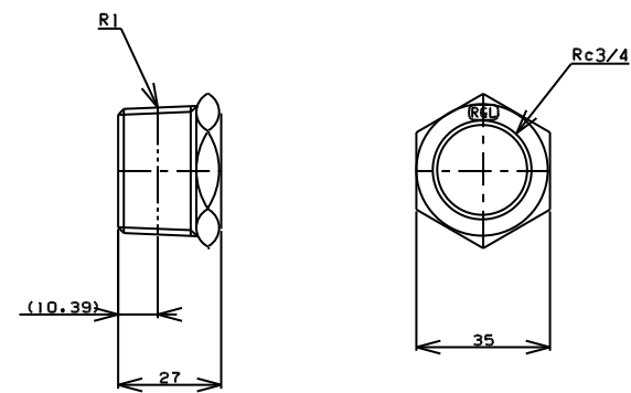
TITLE ブッシング MODEL R-9-1x3/4
