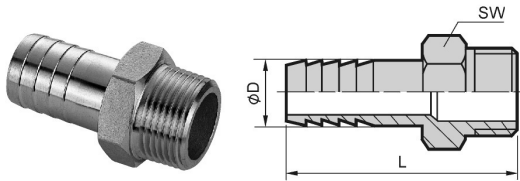
型式:R-7D 単位:mm
