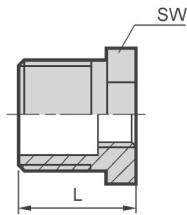
型式:R-9 単位:mm
