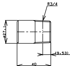
TITLE 片ニップル MODEL R-7C-3/4
