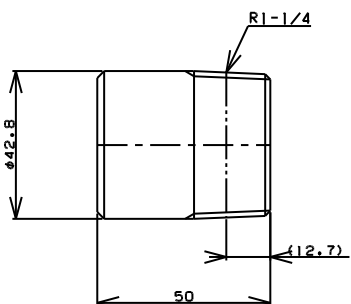
TITLE 片ニップル MODEL R-7C-1-1/4
