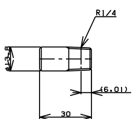
TITLE 片ニップル MODEL R-7C-1/4
