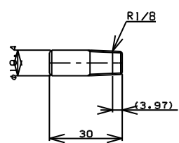
TITLE 片ニップル MODEL R-7C-1/8
