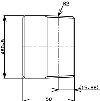
TITLE 片ニップル MODEL R-7C-2
