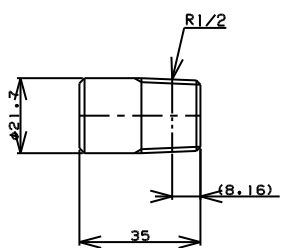
TITLE 片ニップル MODEL R-7C-1/2
