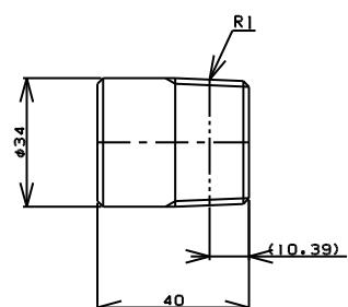
TITLE 片ニップル MODEL R-7C-1
