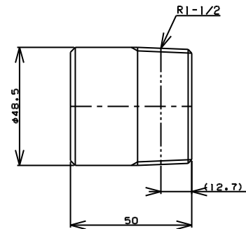
TITLE 片ニップル MODEL R-7C-1-1/2
