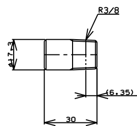
TITLE 片ニップル MODEL R-7C-3/8
