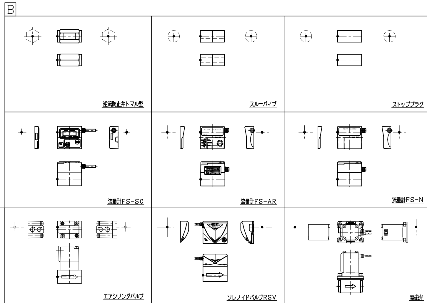
・マジックマニホールドに機器を組み込んだ例
