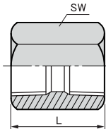
型式:R-12K 単位:mm
