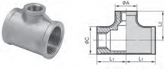
型式:R-2A 単位:mm
