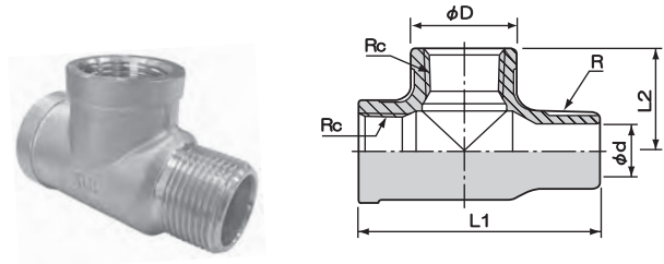
型式:R-2E 単位:mm
