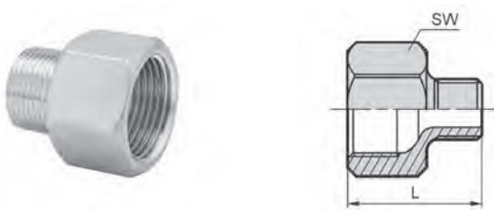
型式:R-9A 単位:mm
